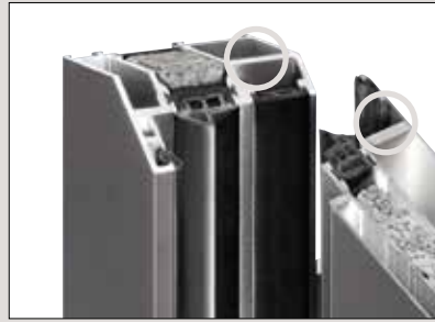
Wandungsstärke bis 3 mm bietet einen sicheren Halt für Schloss und Bandbolzen, Profil verwindungsfest
